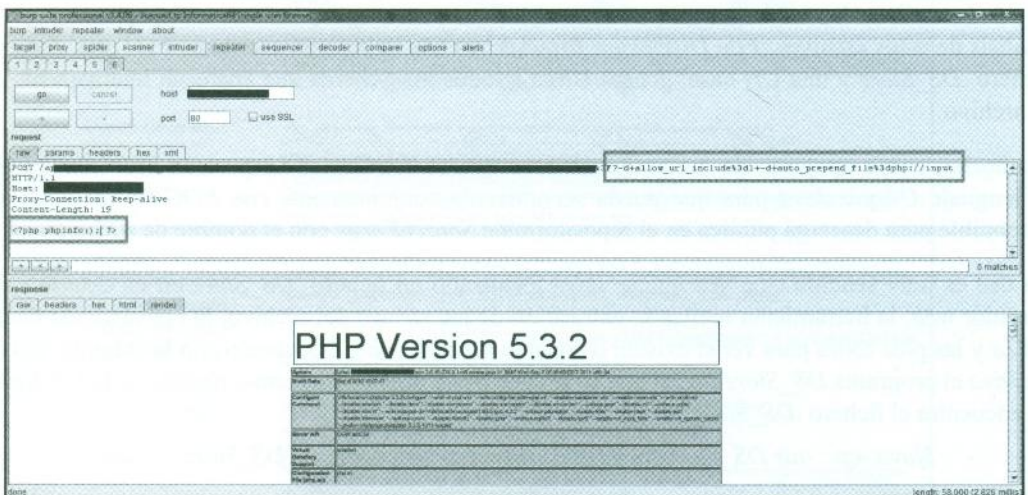
Imagen 04.10: Servidor vulnerable al bug PHP CGI Code Execution .
