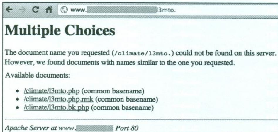
Imagen 04.20: Servidor web con la opción mod_negotiation activa.
